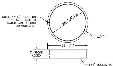
DETAIL F-F SCALE: 1"=1'-0"
