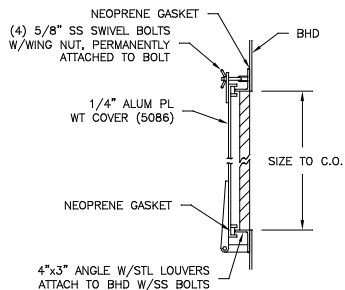
DETAIL D-D SCALE: NONE
